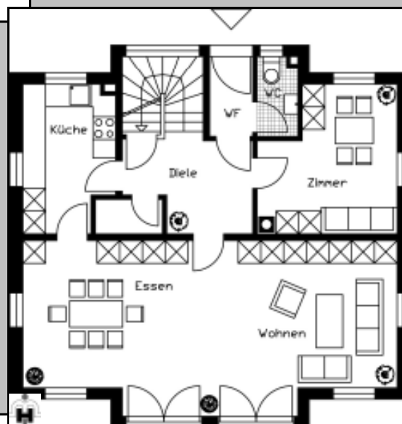
Grundriss Erdgeschoss
