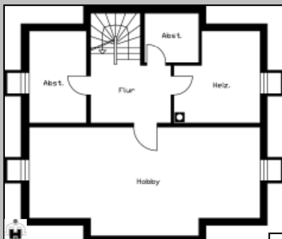
Grundriss Untergeschoss
