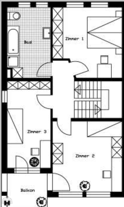
Grundriss Obergeschoss
