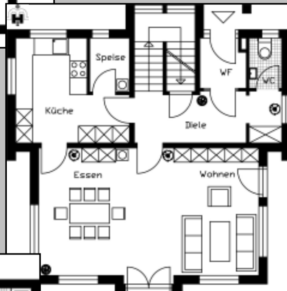
Grundriss Erdgeschoss
