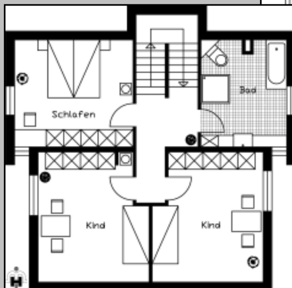
Grundriss Obergeschoss
